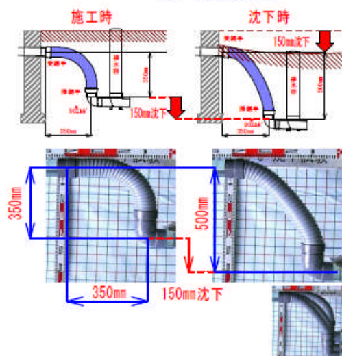
タイシンチンカ (TFJ-75-5) 標準仕様の沈下予測施工仕様
