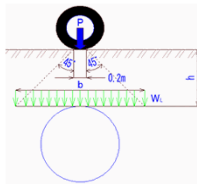
後輪荷重
