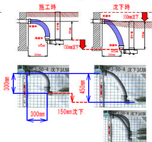
タイシンチンカ (TFJ-50-4) 標準仕様の沈下予測施工仕様
