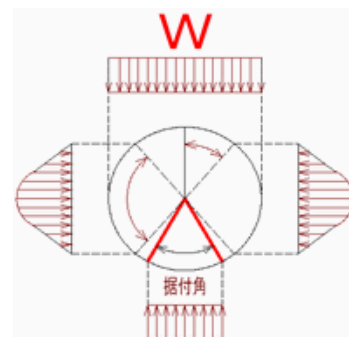
土圧分布
