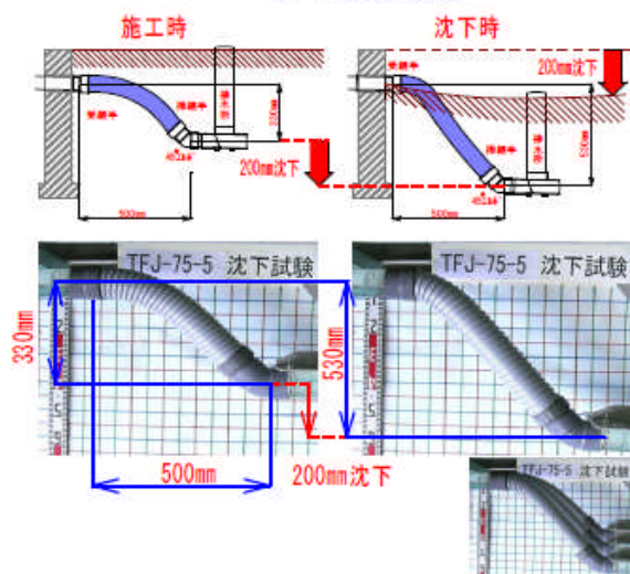
タイシンチンカ (TFJ-75-5) 標準仕様の沈下予測施工仕様
