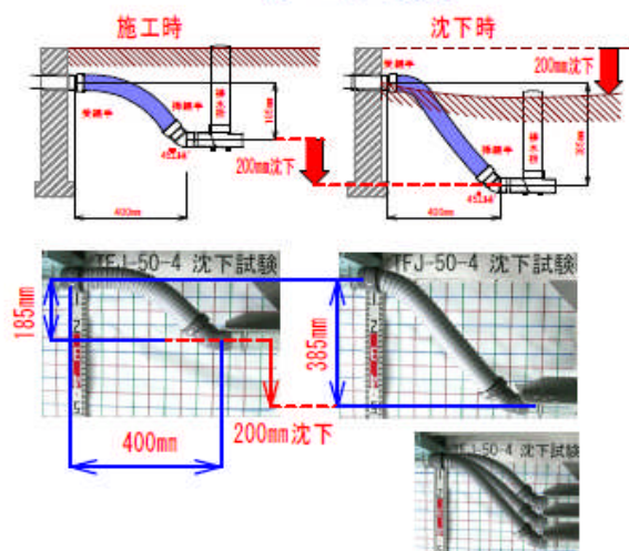
タイシンチンカ (TFJ-50-4) 標準仕様の沈下予測施工仕様
